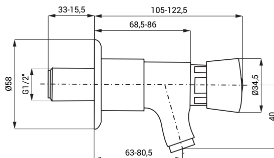
SLT 113U 09014 Nástěnná umyvadlová samouzavírací baterie
