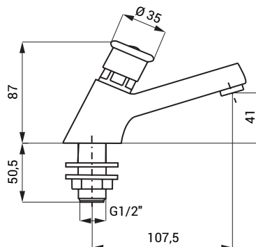
SLT 100U 09000 Stojánková umyvadlová samouzavírací baterie
