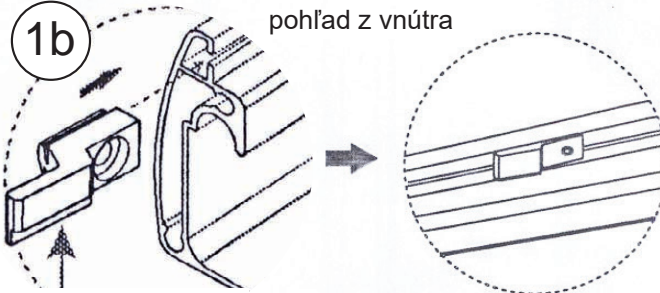
spodný plastový úchyt pevného skla
